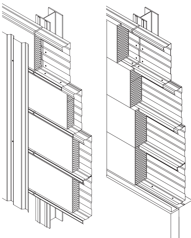
Klasická kazetová stěna a kazetová stěna s předsazeným pláštěm
