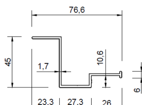
Hliníkový Z profil 10236
