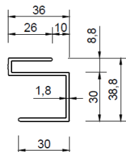
Hliníkový S profil 10235/26
