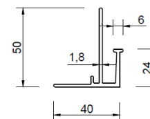
Hliníkový základací profil 10237
