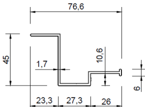
Hliníkový Z profil 10236
