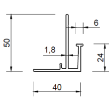
Hliníkový základací profil 10237
