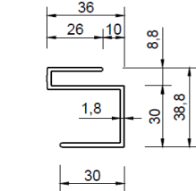
Hliníkový S profil 10235/26
