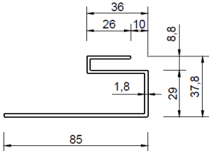
Hliníkový SL profil xx/26
