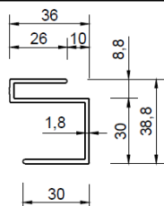
Hliníkový S profil 10235/26
