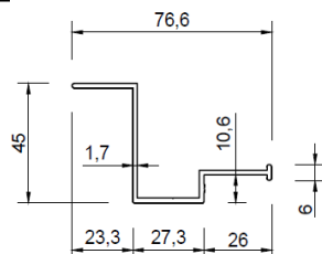
Hliníkový Z profil 10236
