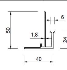
Hliníkový zakládací profil 10237
