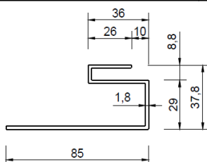
Hliníkový SL profil xx/26
