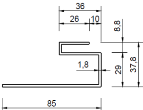
Hliníkový "SL" profil xx/26 Spodní závěsný "S" profil, pro lepení i nýtování
