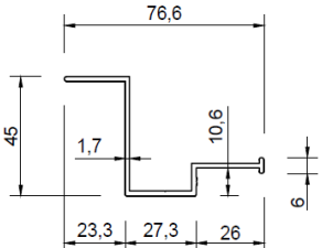
AL "Z" profil 10236 Horní závěsný "Z" profil, pro lepení i nýtování
