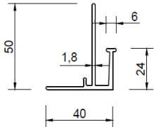
AL základací profil 10237 Zakládací profil
