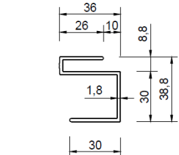
Hliníkový "S" profil 10235/26 Spodní závěsný "S" profil, pro nýtování
